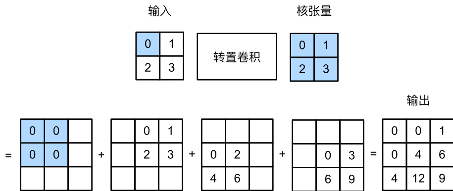
图13.10.1: 卷积核为 2 \times 2 的转置卷积。阴影部分是中间张量的一部分，也是用于计算的输入和卷积核张量元素。
