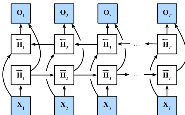
图9.4.2: 双向循环神经网络架构
