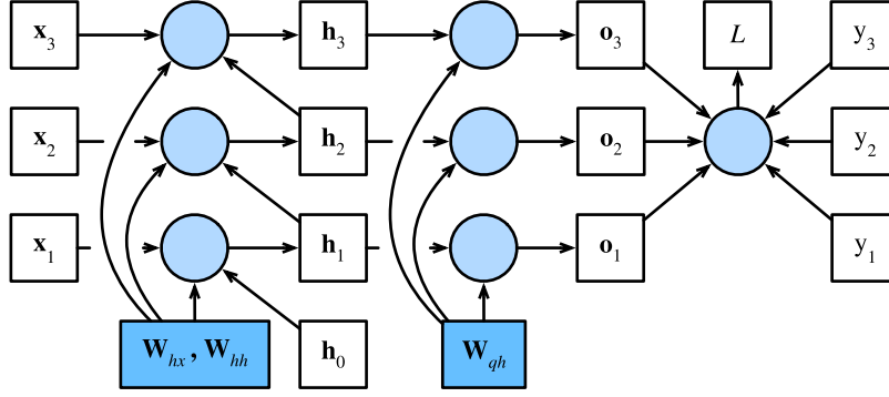
图8.7.2: 上图表示具有三个时间步的循环神经网络模型依赖关系的计算图。未着色的方框表示变量，着色的方框表示参数，圆表示运算符
