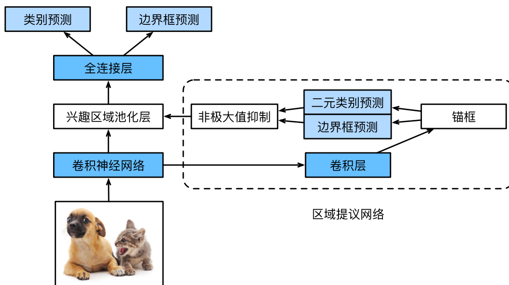
图13.8.4: Faster R-CNN 模型
