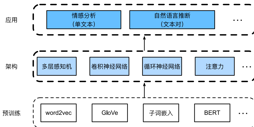
图15.1: 预训练文本表示可以通过不同模型架构，放入不同的下游自然语言处理应用（本章重点介绍如何为不同的下游应用设计模型）
