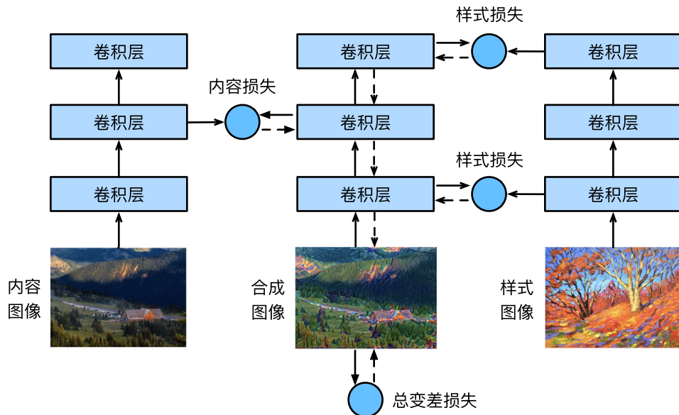
图13.12.2: 基于卷积神经网络的风格迁移。实线箭头和虚线箭头分别表示前向传播和反向传播
