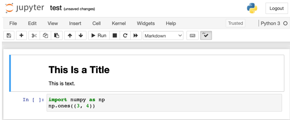
图16.1.2: “test.ipynb” 文件中的markdown和代码块
