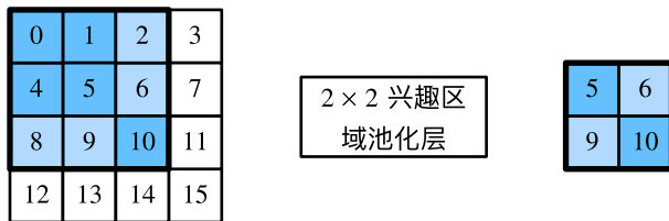
图13.8.3: 一个 2 \times 2 的兴趣区域汇聚层
