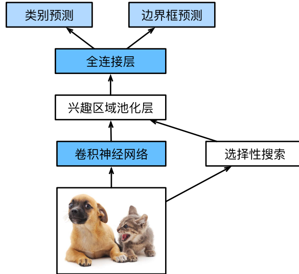
图13.8.2: Fast R-CNN模型
