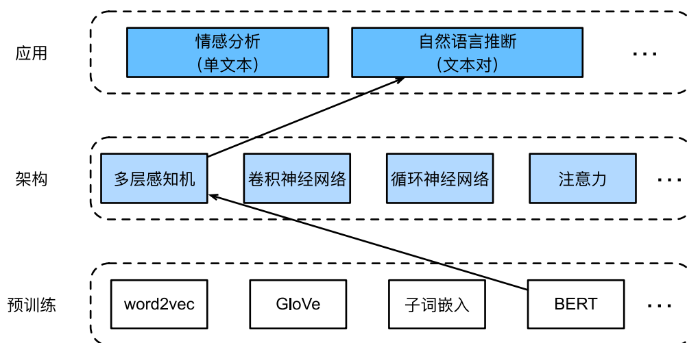
图15.7.1: 将预训练BERT提供给基于多层感知机的自然语言推断架构
