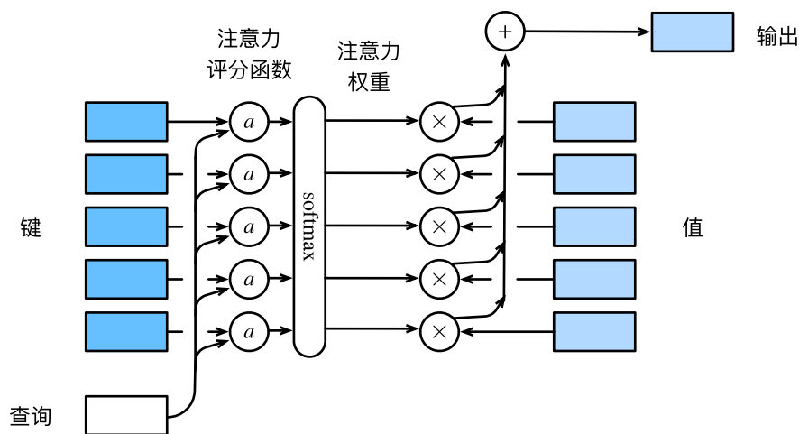
图10.3.1: 计算注意力汇聚的输出为值的加权和
