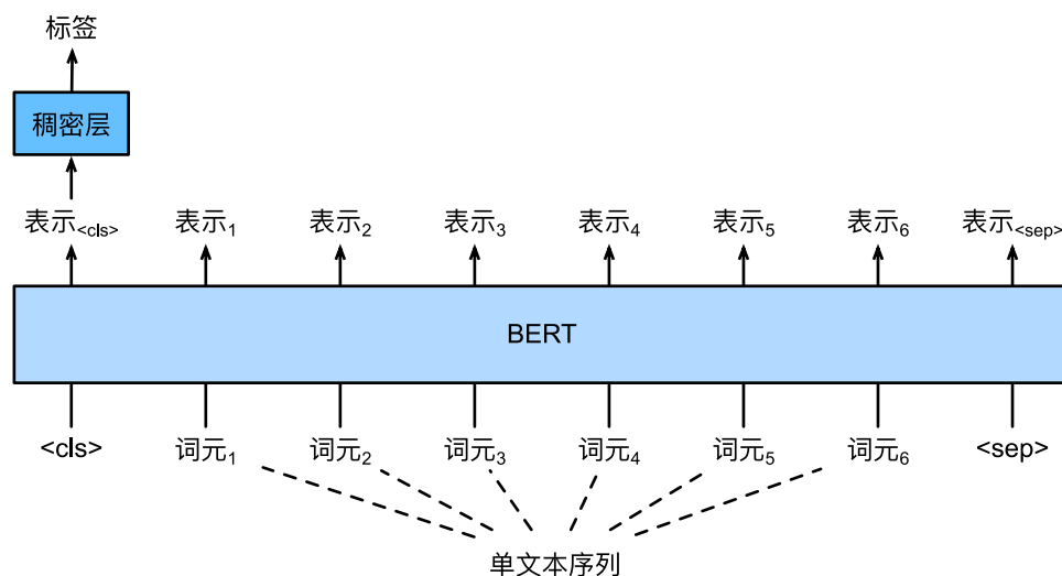
图15.6.1: 微调BERT用于单文本分类应用，如情感分析和测试语言可接受性（这里假设输入的单文本有六个词元）
