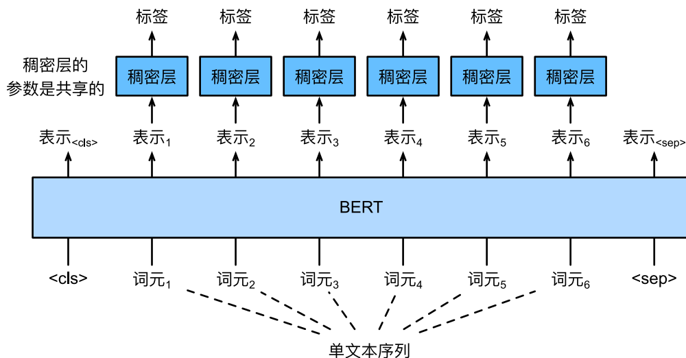
图15.6.3: 文本标记应用的BERT微调，如词性标记。假设输入的单个文本有六个词元。
