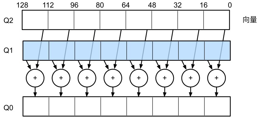
图12.4.5: 128位NEON矢量化
