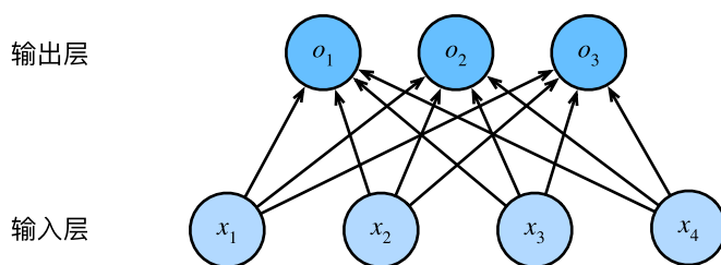
图3.4.1: softmax回归是一种单层神经网络
