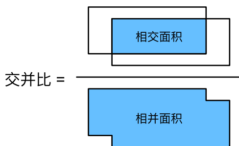
图13.4.1: 交并比是两个边界框相交面积与相并面积之比。
