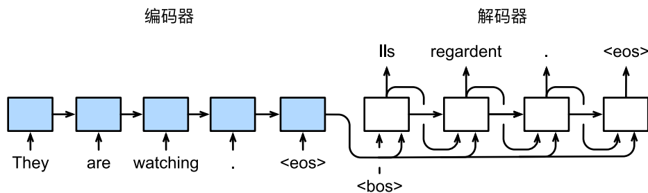
图9.7.3: 使用循环神经网络编码器-解码器逐词元地预测输出序列。
