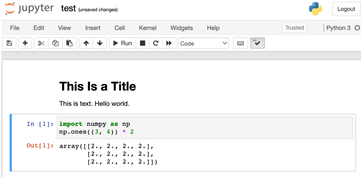
图16.1.7: 运行代码单元格以获得输出
