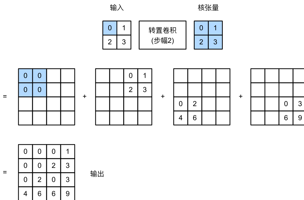
图13.10.2: 卷积核为2 × 2，步幅为2的转置卷积。阴影部分是中间张量的一部分，也是用于计算的输入和卷积核张量元素。
