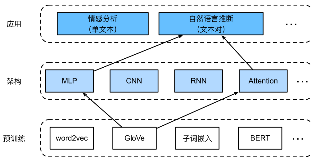
图15.5.1: 将预训练GloVe送入基于注意力和MLP的自然语言推断架构
