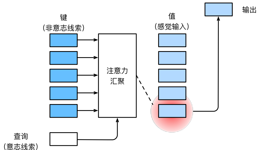
图10.1.3: 注意力机制通过注意力汇聚将查询（自主性提示）和键（非自主性提示）结合在一起，实现对值（感官输入）的选择倾向
