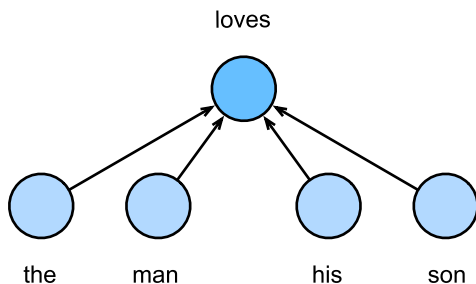
图14.1.2: 连续词袋模型考虑了给定周围上下文词生成中心词条件概率
