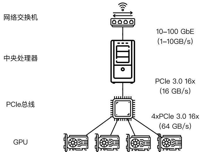
图12.7.2: 一个4路GPU服务器
