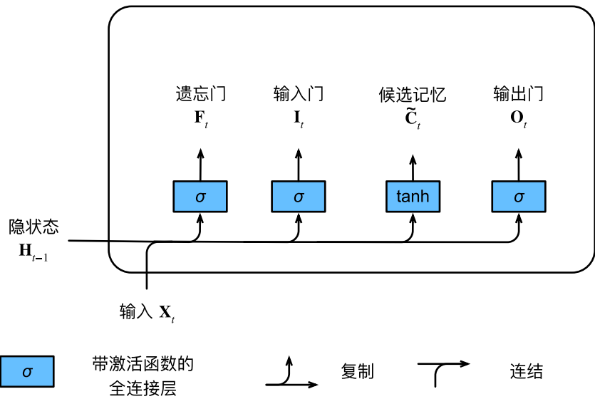
图9.2.2: 长短期记忆模型中的候选记忆元
