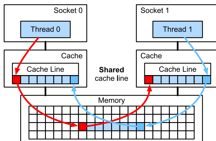
图12.4.6: 错误共享（图片由英特尔提供）
