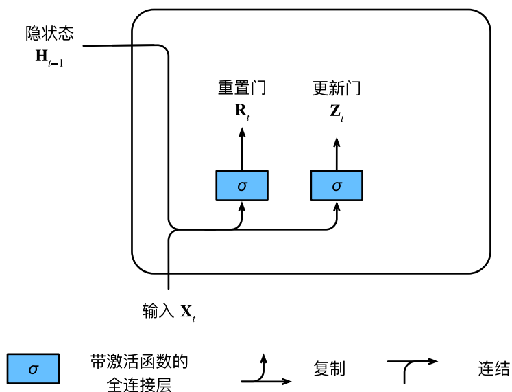
图9.1.1: 在门控循环单元模型中计算重置门和更新门
