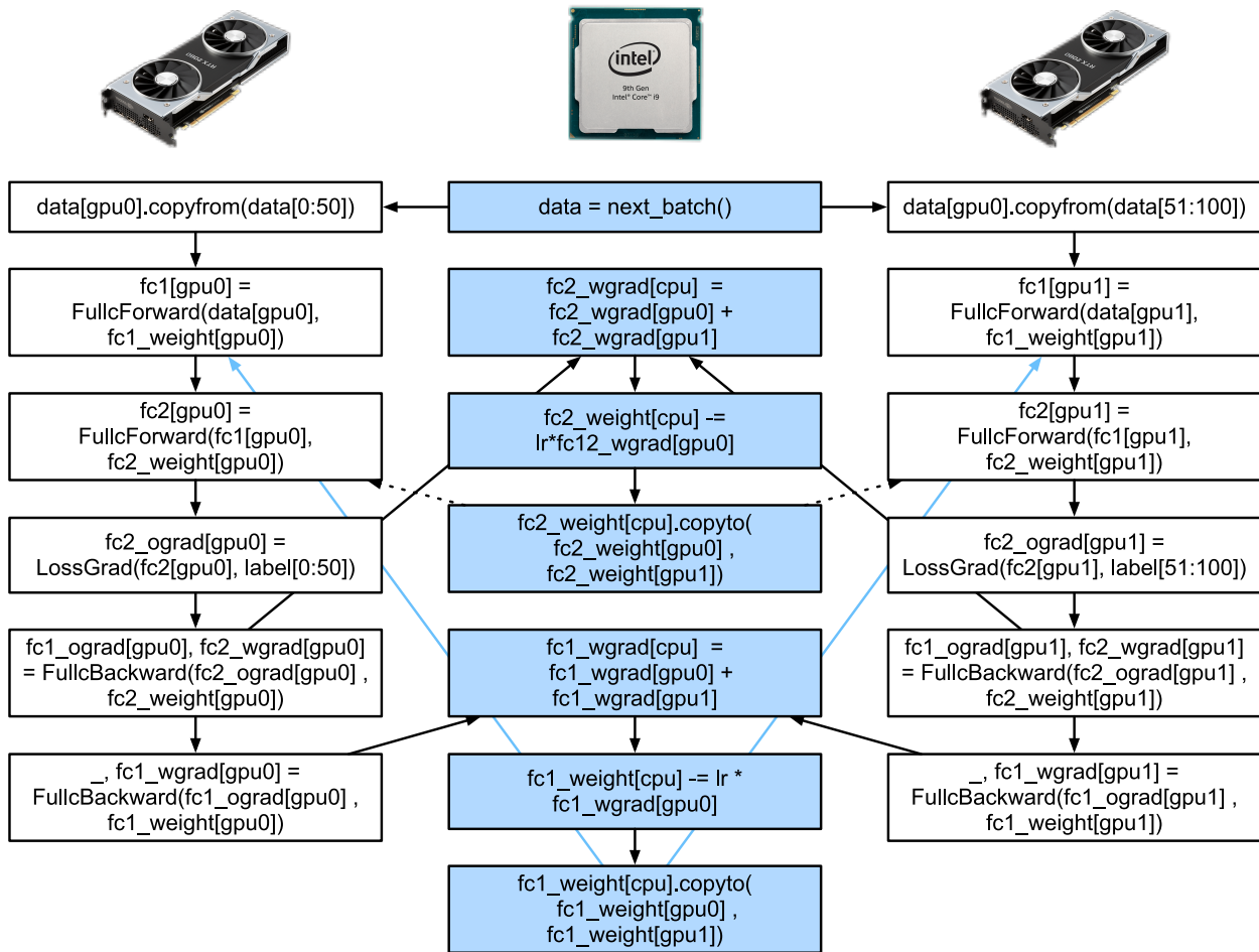
图12.3.1: 在一个CPU和两个GPU上的两层的多层感知机的计算图及其依赖关系
