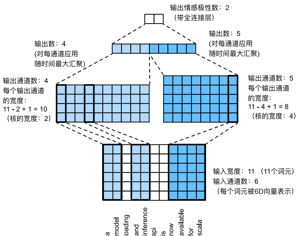
图15.3.5: textCNN的模型架构
