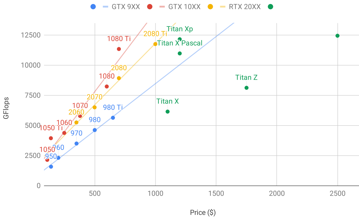
图16.4.1: 浮点计算能力和价格比较
