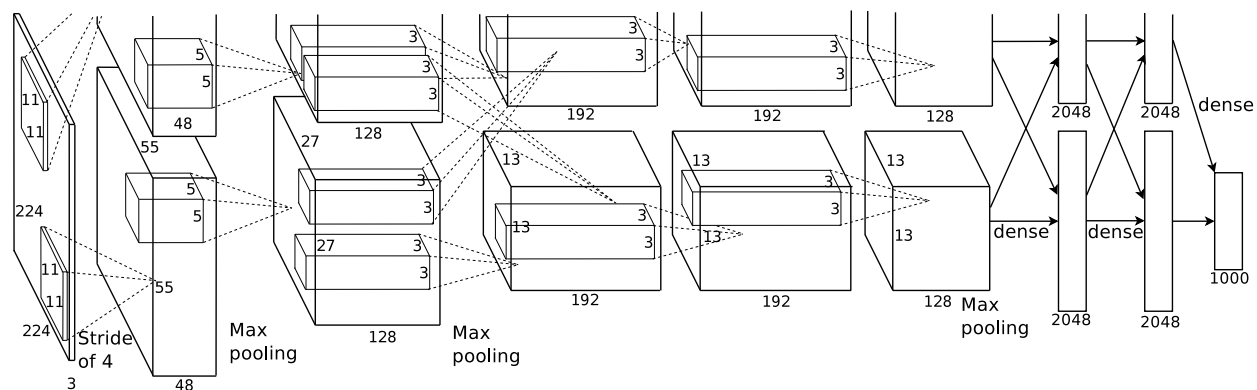
图12.5.1: 由于GPU显存有限, 原有AlexNet设计中的模型并行
