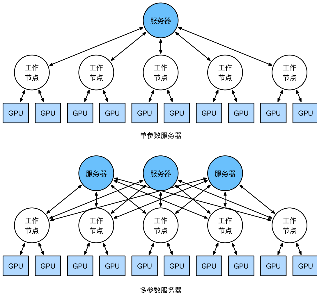
图12.7.8: 上图: 单参数服务器是一个瓶颈, 因为它的带宽是有限的; 下图: 多参数服务器使用聚合带宽存储部分参数
