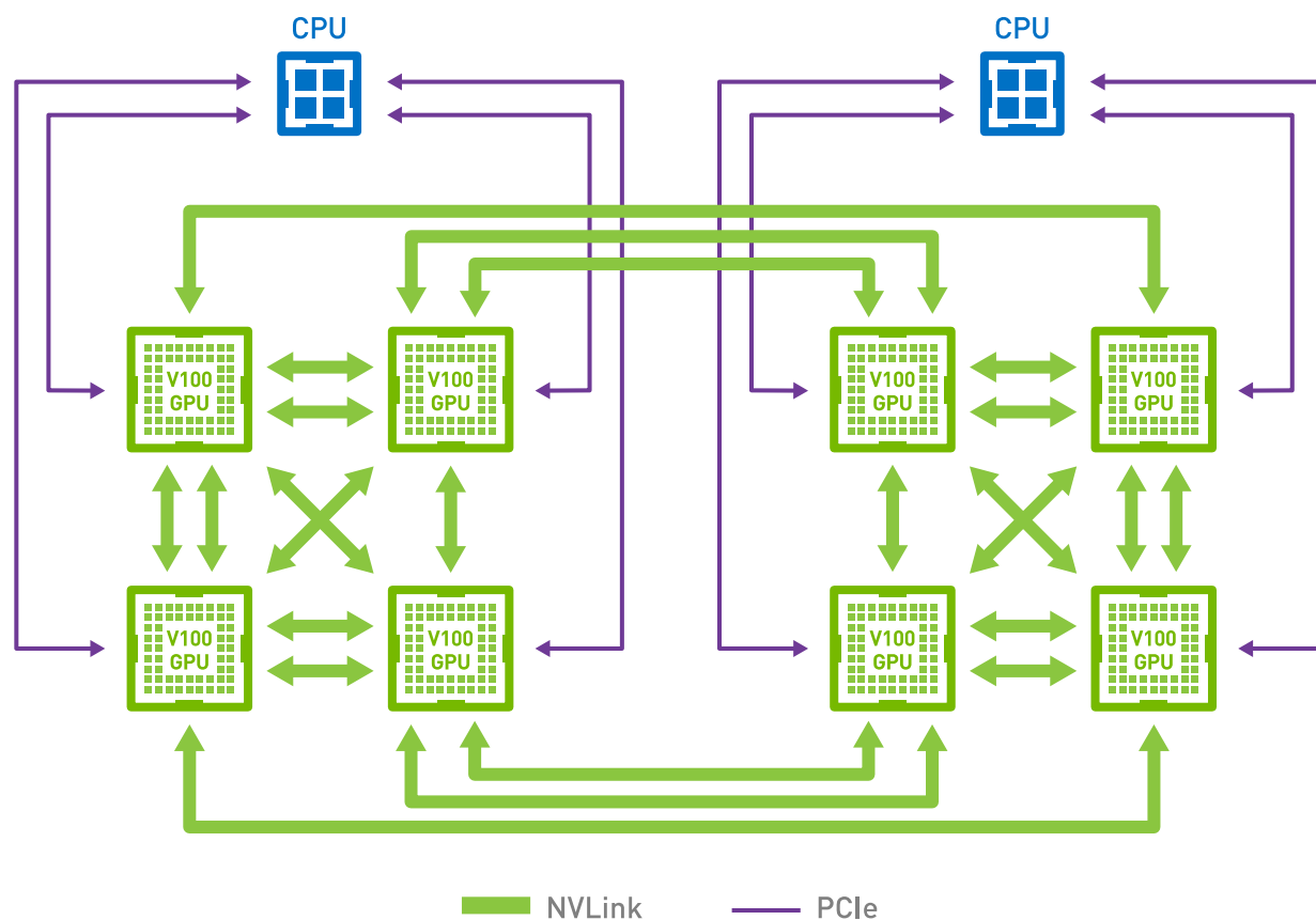
图12.7.4: 在8台V100 GPU服务器上连接NVLink (图片由英伟达提供)
