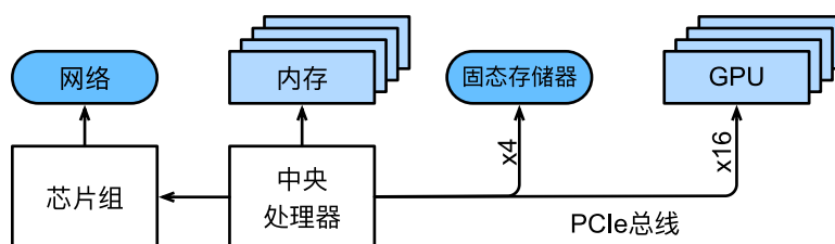
图12.4.2: 计算机组件的连接
