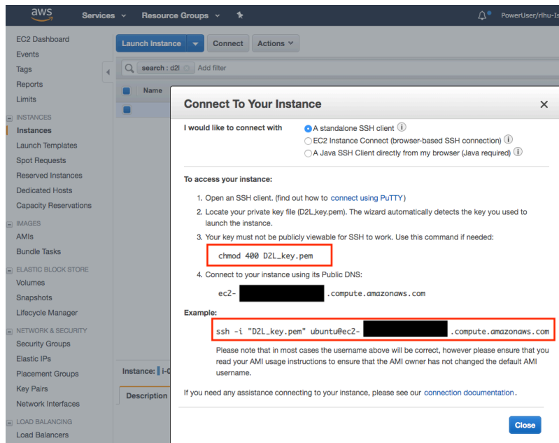
图16.3.10: 查看实例访问和启动方法
