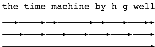
图8.7.1: 比较RNN中计算梯度的策略, 3行自上而下分别为: 随机截断、常规截断、完整计算
