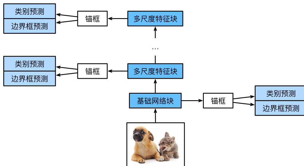
图13.7.1: 单发多框检测模型主要由一个基础网络块和若干多尺度特征块串联而成。
