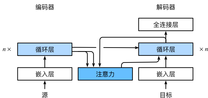
图10.4.1: 一个带有Bahdanau注意力的循环神经网络编码器-解码器模型
