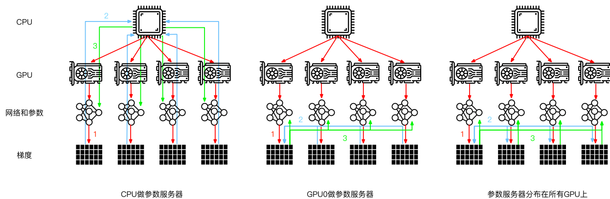
图12.7.3: 参数同步策略
