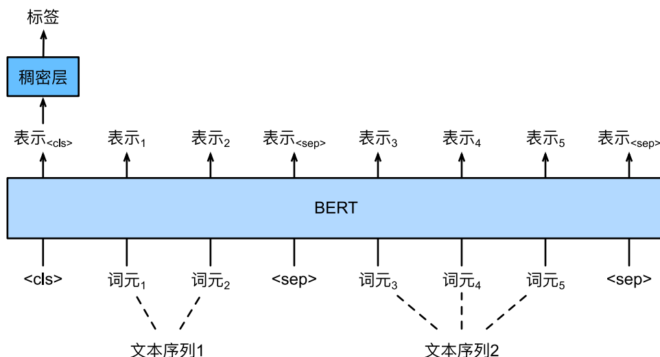
图15.6.2: 文本对分类或回归应用的BERT微调，如自然语言推断和语义文本相似性（假设输入文本对分别有两个词元和三个词元）
