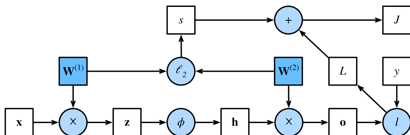
图4.7.1: 前向传播的计算图
