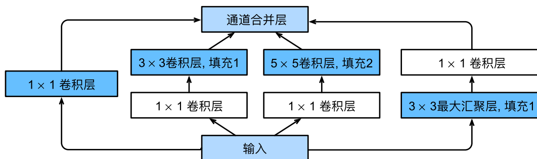
图7.4.1: Inception块的架构。
