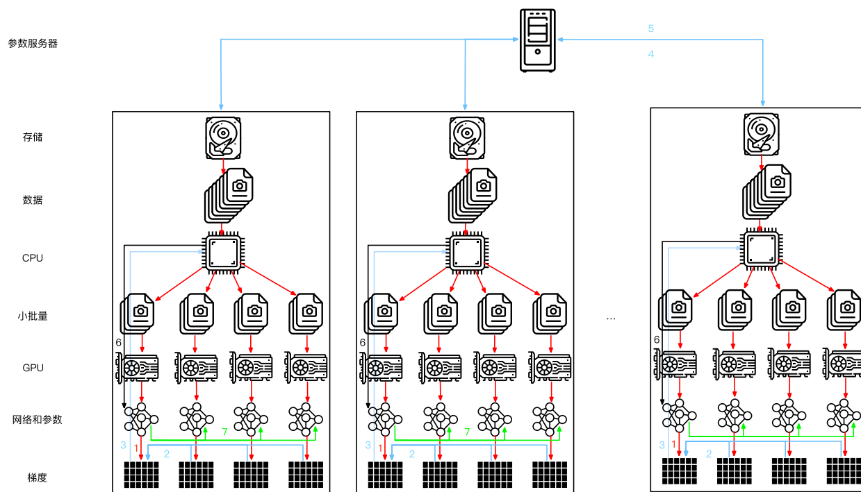
图12.7.7: 多机多GPU分布式并行训练
