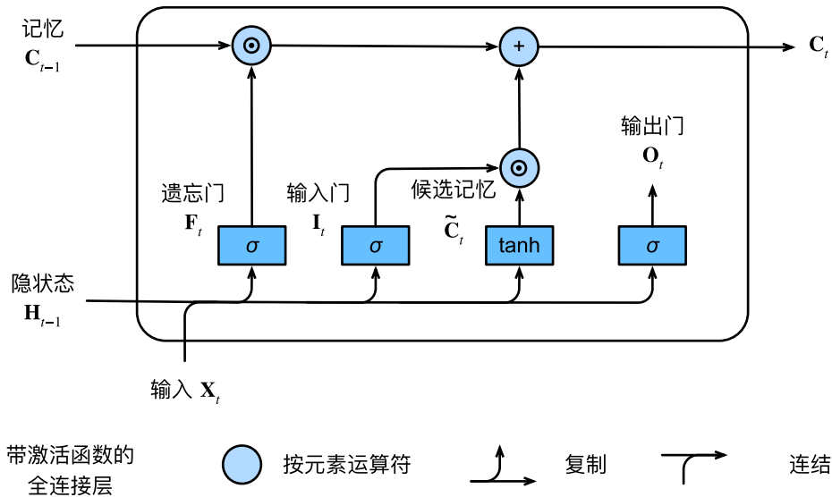
图9.2.3: 在长短期记忆网络模型中计算记忆元
