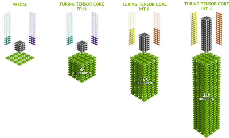
图12.4.9: NVIDIA Turing架构中的张量核心 (图片由英伟达提供)
