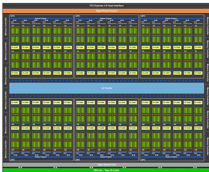
图12.4.8: NVIDIA Turing架构 (图片由英伟达提供)
