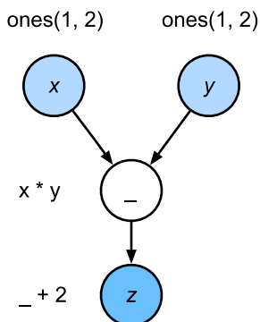
图12.2.2: 后端跟踪计算图中各个步骤之间的依赖关系
