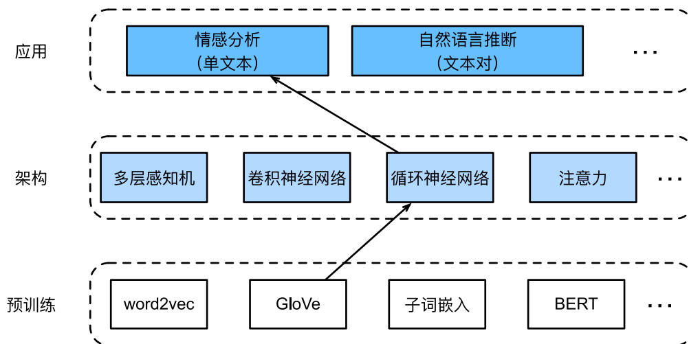
图15.2.1: 将GloVe送入基于循环神经网络的架构，用于情感分析
