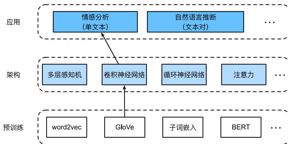
图15.3.1: 将GloVe放入卷积神经网络架构进行情感分析
