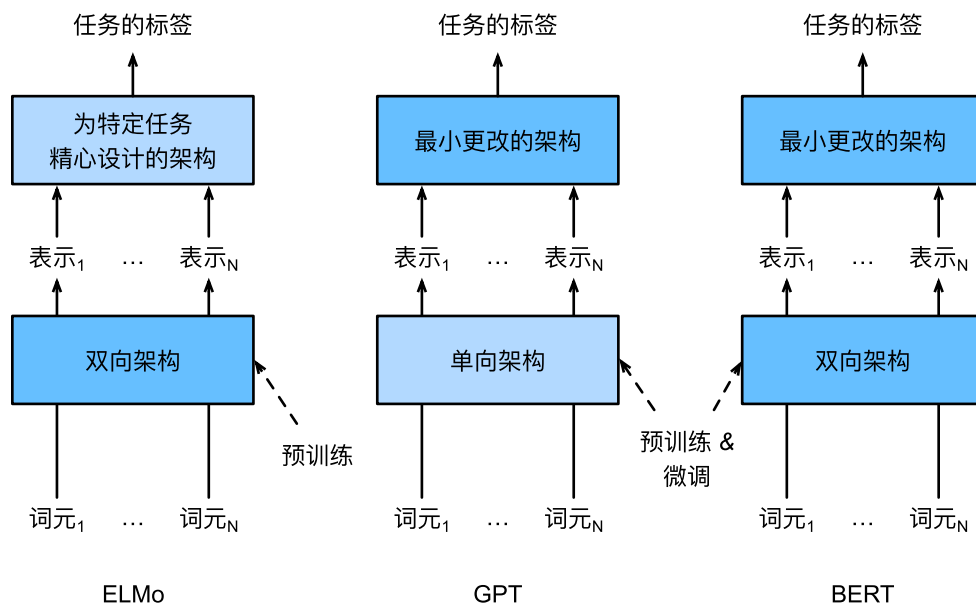
图14.8.1: ELMo、GPT和BERT的比较
