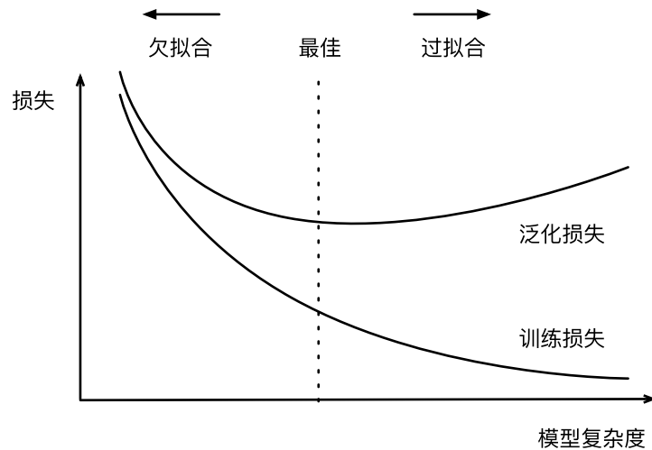
图4.4.1: 模型复杂度对欠拟合和过拟合的影响
