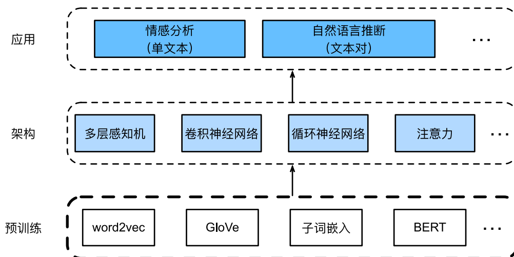
图14.1: 预训练好的文本表示可以放入各种深度学习架构，应用于不同自然语言处理任务（本章主要研究上游文本的预训练）
