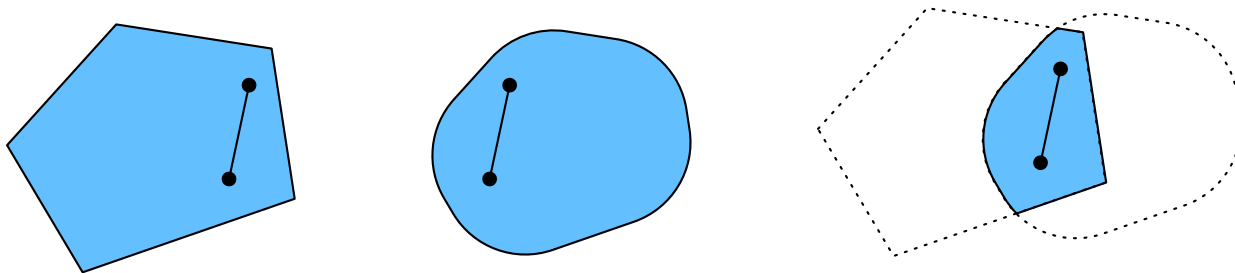
图11.2.2: 两个凸集的交集是凸的。
