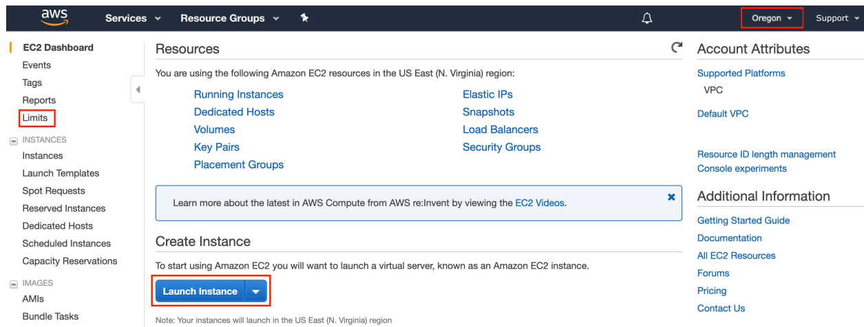
图16.3.2: EC2面板
