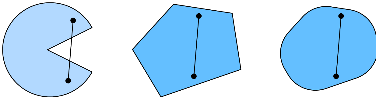
图11.2.1: 第一组是非凸的, 另外两组是凸的。
