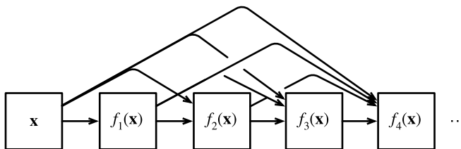
图7.7.2: 稠密连接。
