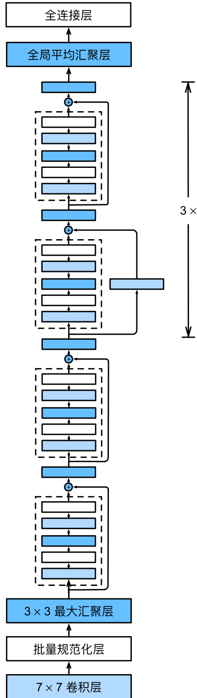
图7.6.4: ResNet-18 架构
