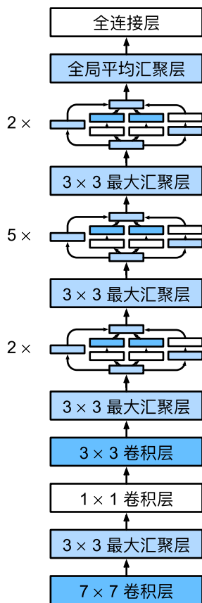
图7.4.2: GoogLeNet架构。
