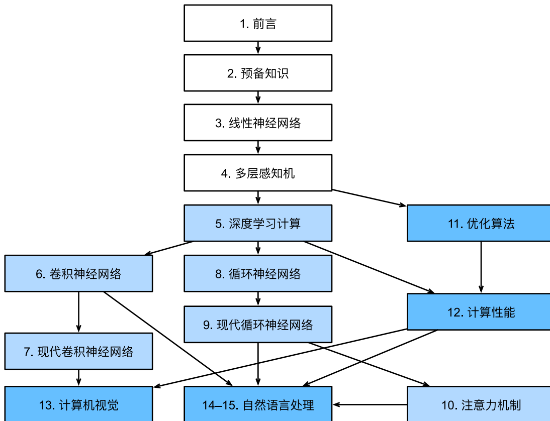
图1: 全书结构
