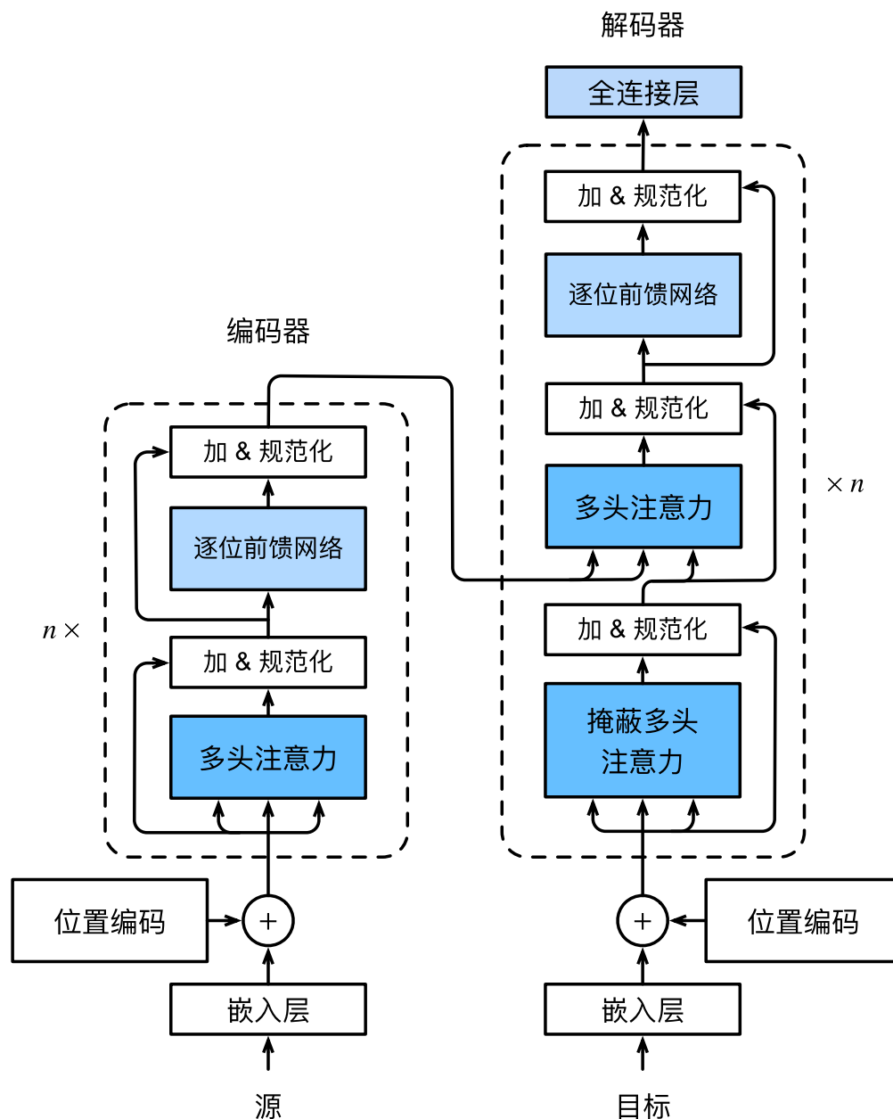
图10.7.1: transformer架构
