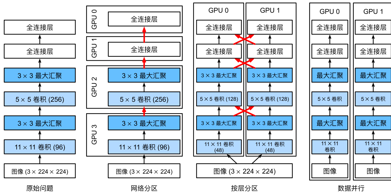
图12.5.2: 在多个GPU上并行化。从左到右：原始问题、网络并行、分层并行、数据并行
