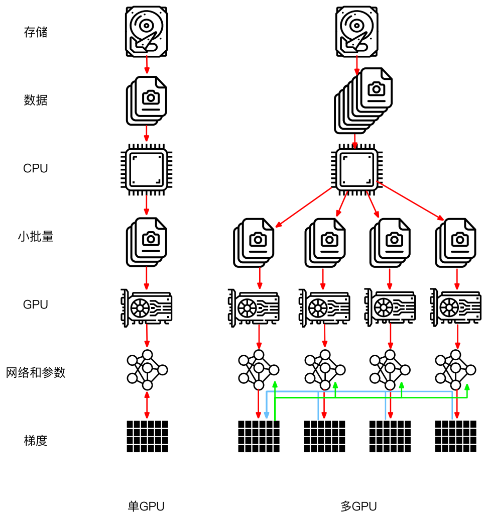
图12.7.1: 左图是单GPU训练；右图是多GPU训练的一个变体：(1) 计算损失和梯度，(2) 所有梯度聚合在一个GPU上，(3) 发生参数更新，并将参数重新广播给所有GPU
