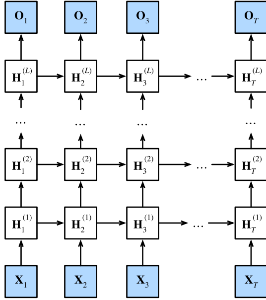
图9.3.1: 深度循环神经网络结构
