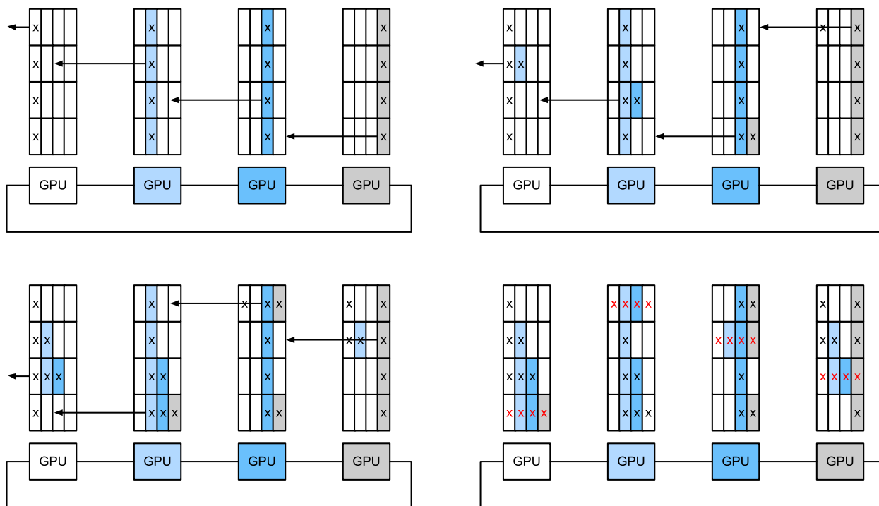
图12.7.6: 跨4个节点的环同步。每个节点开始向其左邻居发送部分梯度，直到在其右邻居中找到聚合的梯度
