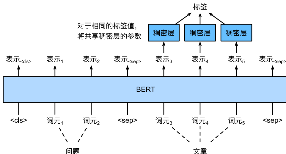
图15.6.4: 对问答进行BERT微调 (假设输入文本对分别有两个和三个词元)
