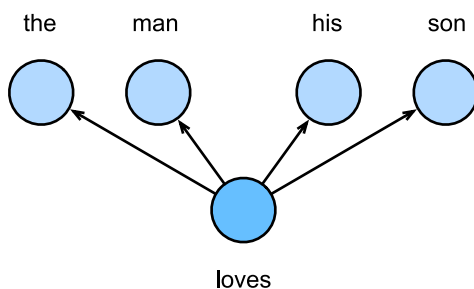
图14.1.1: 跳元模型考虑了在给定中心词的情况下生成周围上下文词的条件概率
