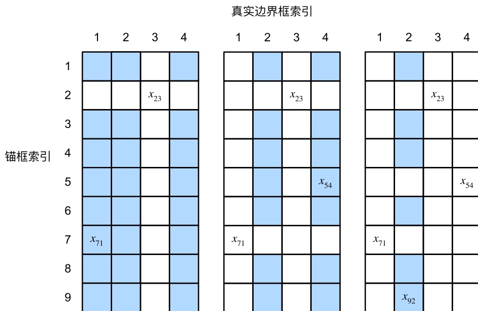
图13.4.2: 将真实边界框分配给锚框。
