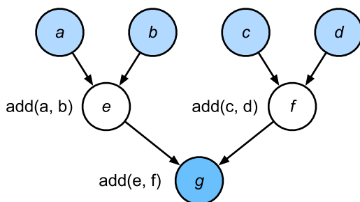
图12.1.1: 命令式编程中的数据流
