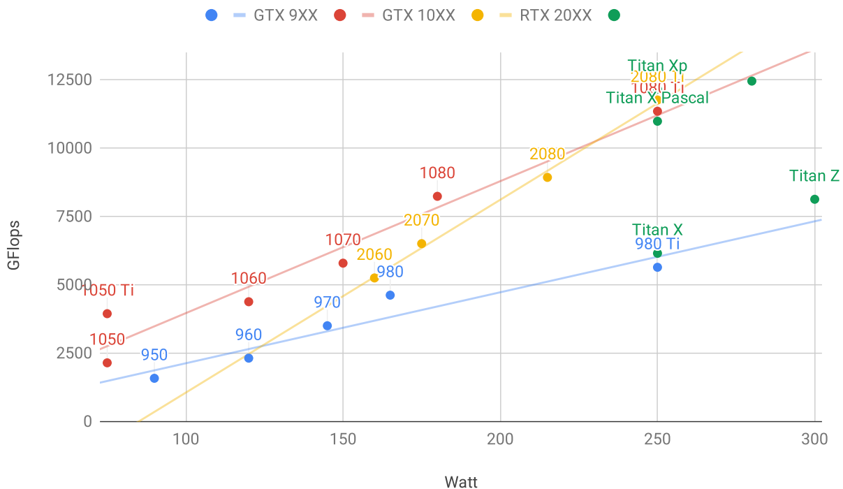
图16.4.2: 浮点计算能力和能耗
