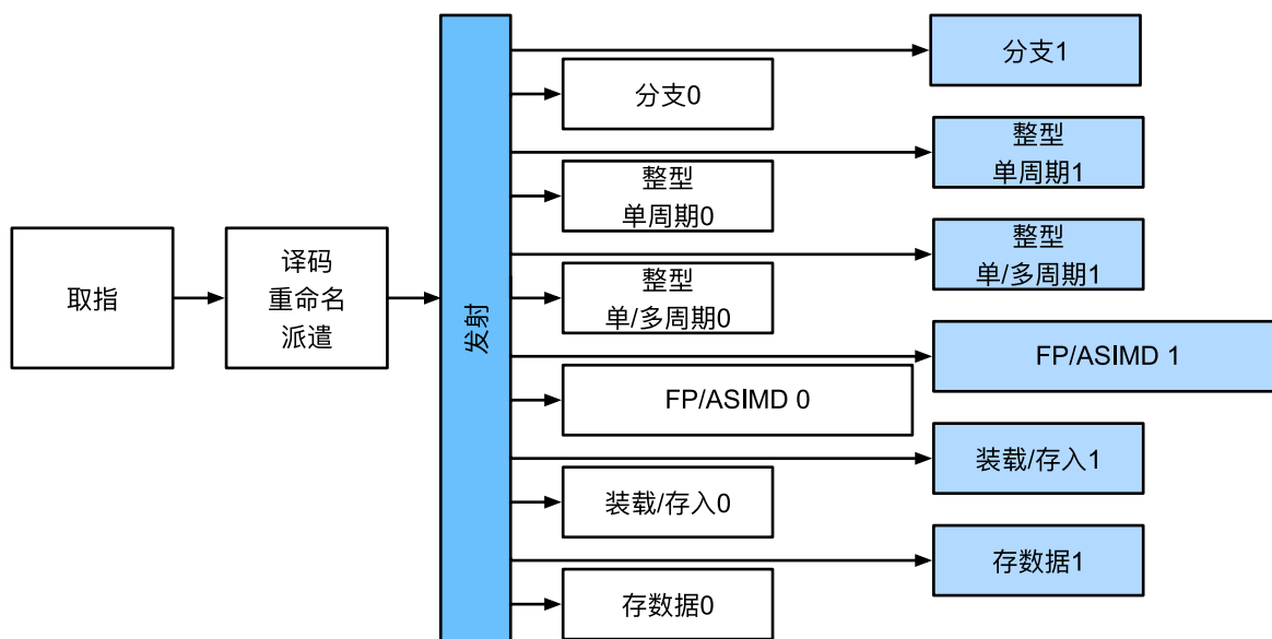
图12.4.4: ARM Cortex A77微体系结构
