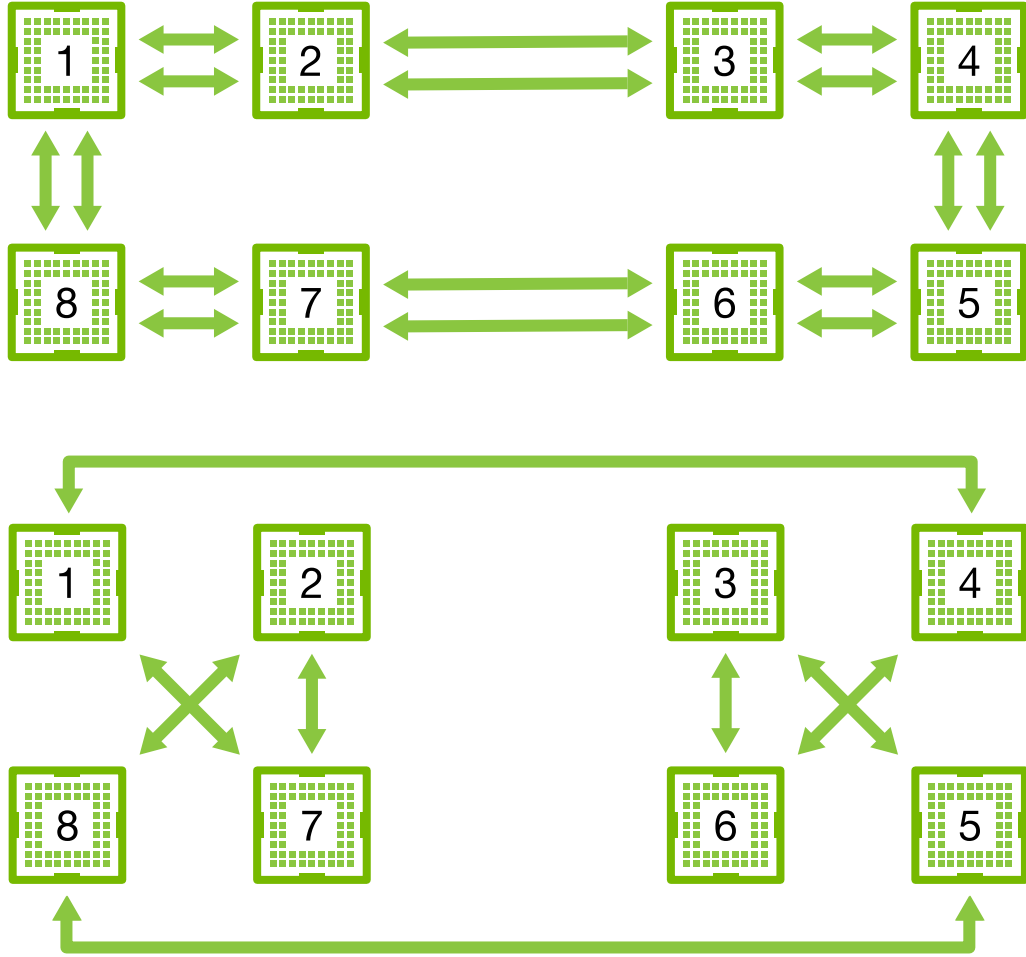
图12.7.5: 将NVLink网络分解为两个环。
