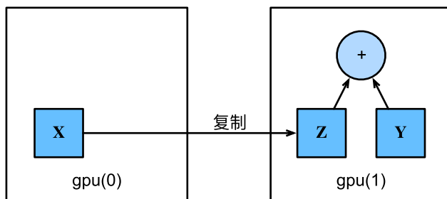
图5.6.1: 复制数据以在同一设备上执行操作
