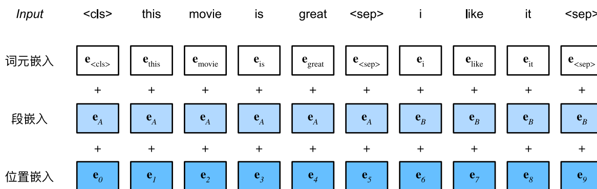
图14.8.2: BERT输入序列的嵌入是词元嵌入、片段嵌入和位置嵌入的和
