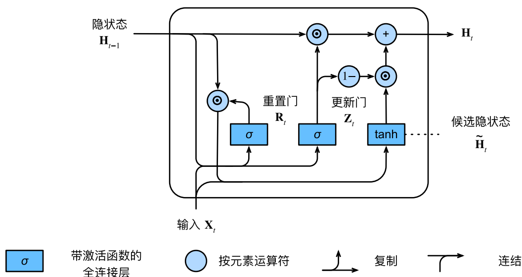
图9.1.3: 计算门控循环单元模型中的隐状态
