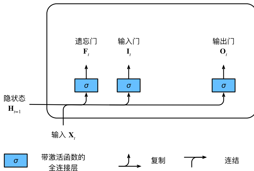
图9.2.1: 长短期记忆模型中的输入门、遗忘门和输出门
