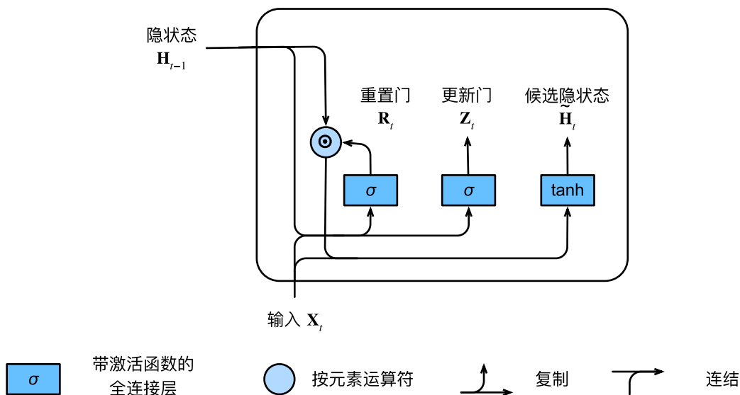
图9.1.2: 在门控循环单元模型中计算候选隐状态
