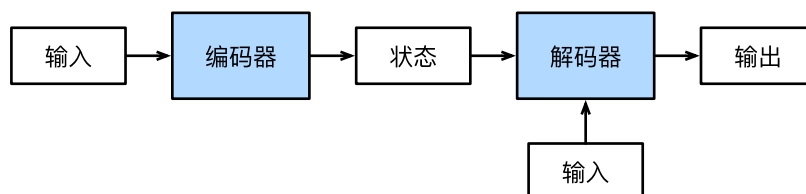
图9.6.1: 编码器-解码器架构
