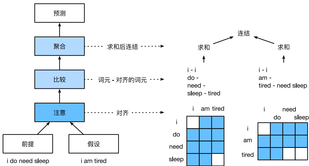
图15.5.2: 利用注意力机制进行自然语言推断
