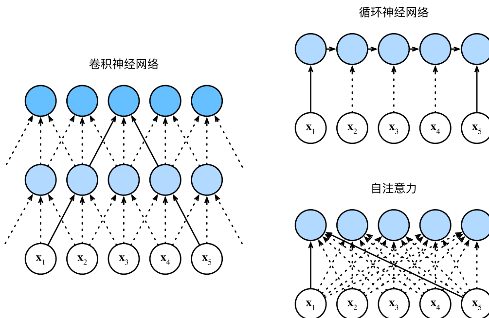
图10.6.1: 比较卷积神经网络（填充词元被忽略）、循环神经网络和自注意力三种架构
