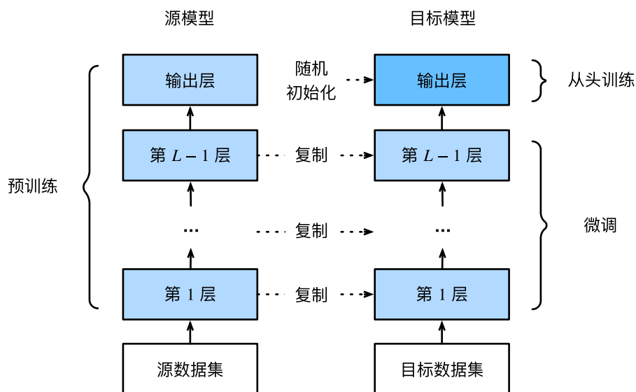
图13.2.1: 微调。
