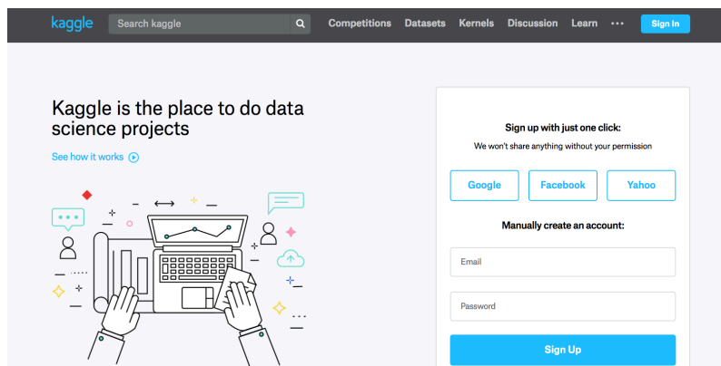
图4.10.1: Kaggle网站
