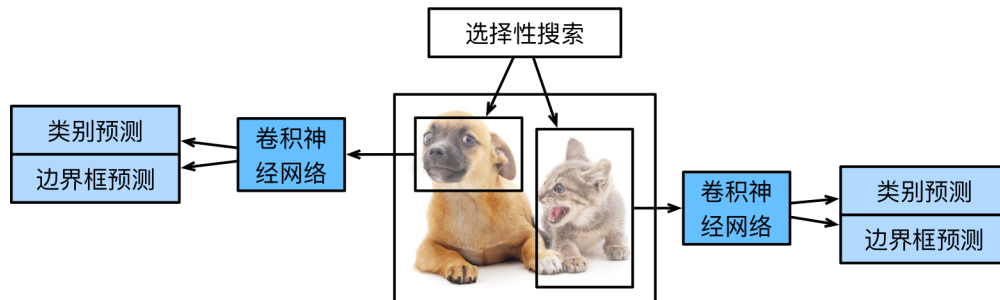
图13.8.1: R-CNN模型
