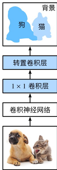
图13.11.1: 全卷积网络
