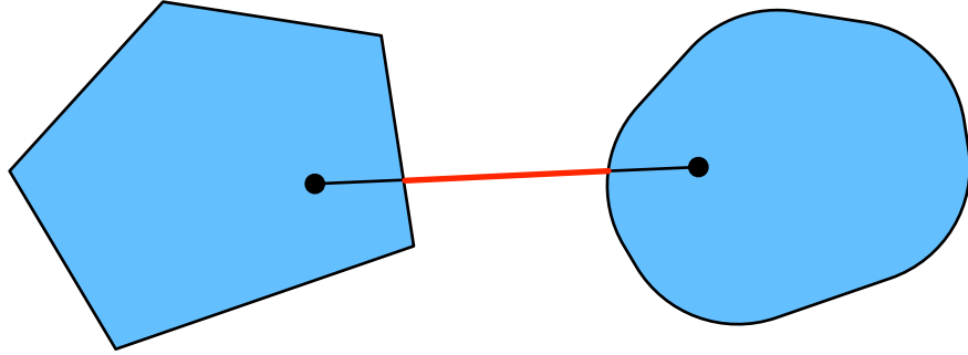
图11.2.3: 两个凸集的并集不一定是凸的。
