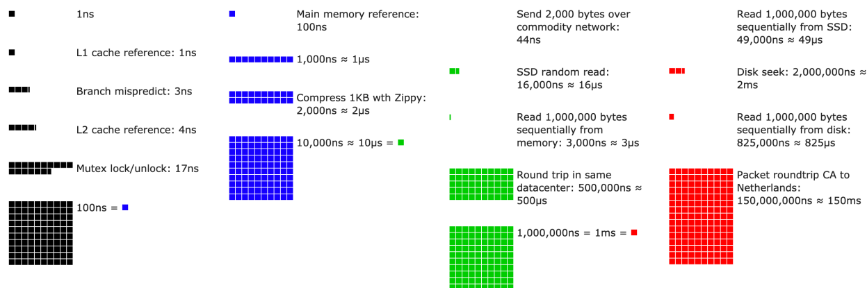
图12.4.1: 每个程序员都应该知道的延迟数字
