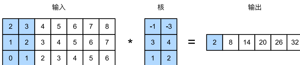
图15.3.4: 具有单个输入通道的二维互相关操作。阴影部分是第一个输出元素以及用于输出计算的输入和内核张量元素: 2 \times (-1) + 3 \times (-3) + 1 \times 3 + 2 \times 4 + 0 \times 1 + 1 \times 2 = 2
