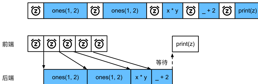
图12.2.3: 前端和后端的交互
