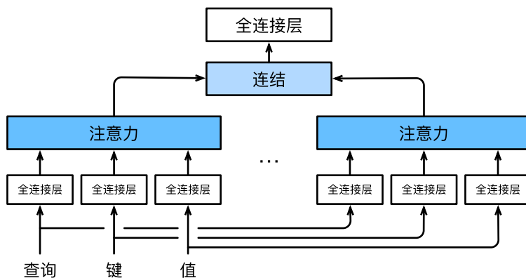
图10.5.1: 多头注意力：多个头连结然后线性变换
