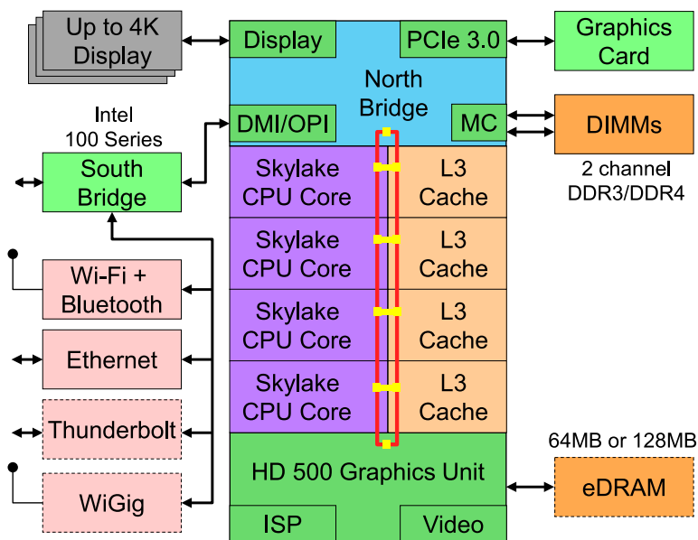
图12.4.3: Intel Skylake消费级四核CPU
