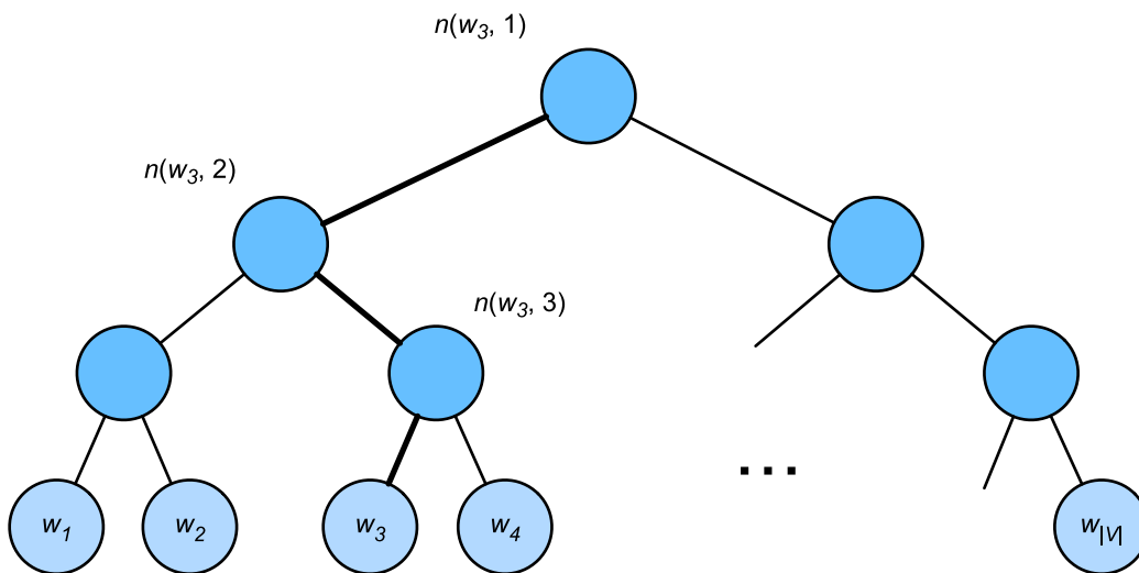
图14.2.1: 用于近似训练的分层softmax, 其中树的每个叶节点表示词表中的一个词
