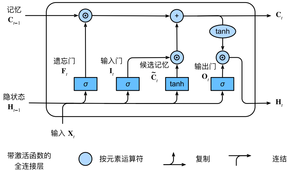
图9.2.4: 在长短期记忆模型中计算隐状态
