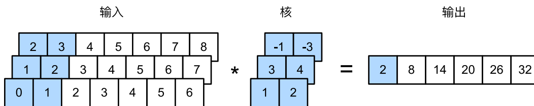
图15.3.3: 具有3个输入通道的一维互相关运算。阴影部分是第一个输出元素以及用于输出计算的输入和核张量元素: 2 \times (-1) + 3 \times (-3) + 1 \times 3 + 2 \times 4 + 0 \times 1 + 1 \times 2 = 2
