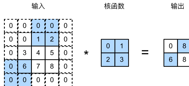
图6.3.2: 垂直步幅为 3，水平步幅为 2 的二维互相关运算。
