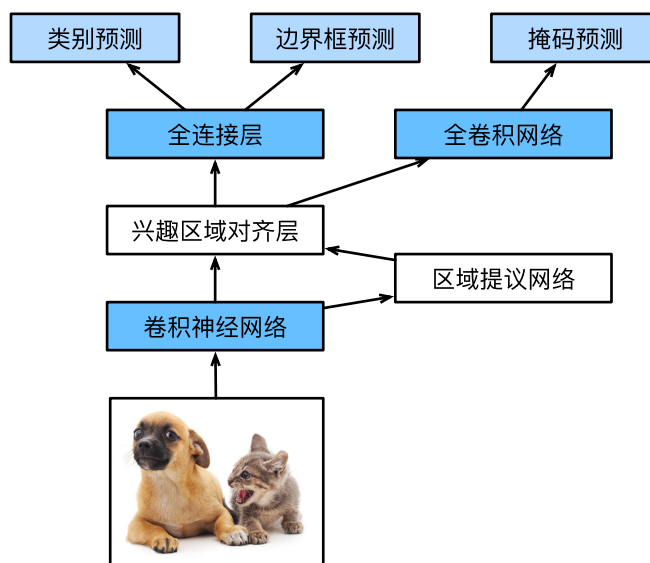
图13.8.5: Mask R-CNN 模型
